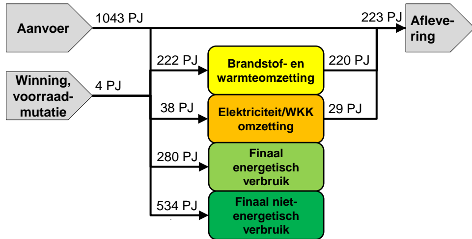
Figuur 1: Energiebalans voor de chemische industrie in 2009. Bron: (CBS, 2012c) 1
