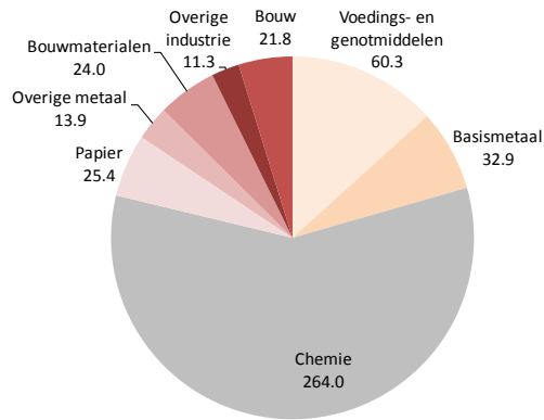
Figuur 10: Finaal thermisch verbruik naar industriesector [PJ]
